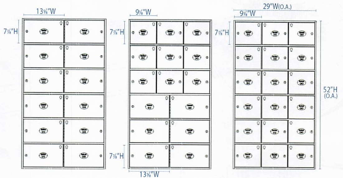
12 DOOR INSERT
